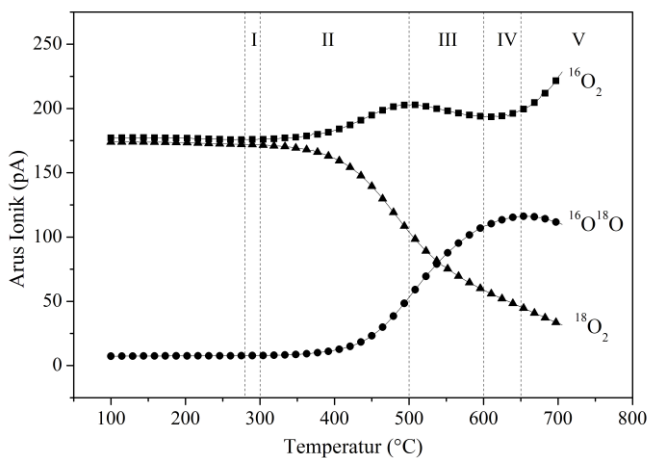
Gambar 1 Pertukaran isotop oksigen gas dan oksigen dalam patatan katalis perovskit. Biasakan untuk menunjukkan signifikansi dari gambar pada judul gambar ( caption ). Sumber: Shahab, Sumaryo, Usman, n.d., p. 3
